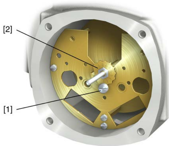
рис. 84: Блок управления с согласующим редуктором
