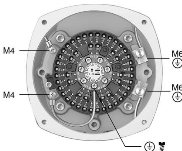
рис. 35: Контакты заземления в соединительном каркасе
