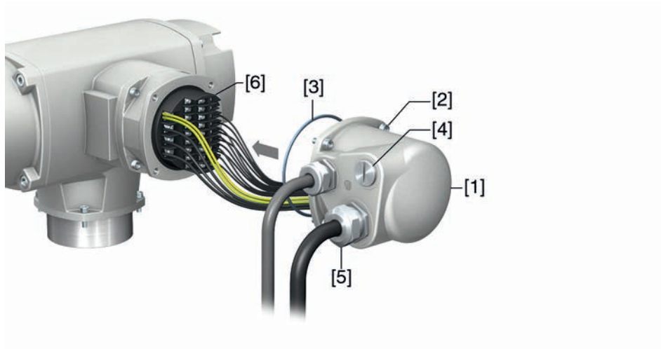
рис. 24: Порядок закрытия отсека контактов
