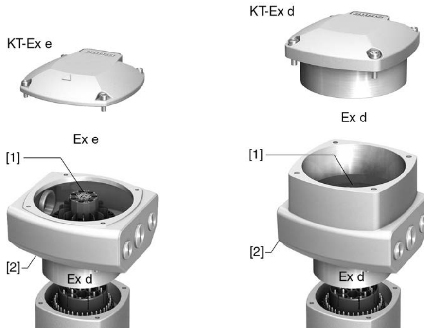
рис. 31: Электрическое подключение КТ/КМ
