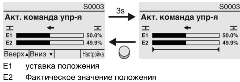
рис. 62: Индикация при управлении уставкой (позиционер)
