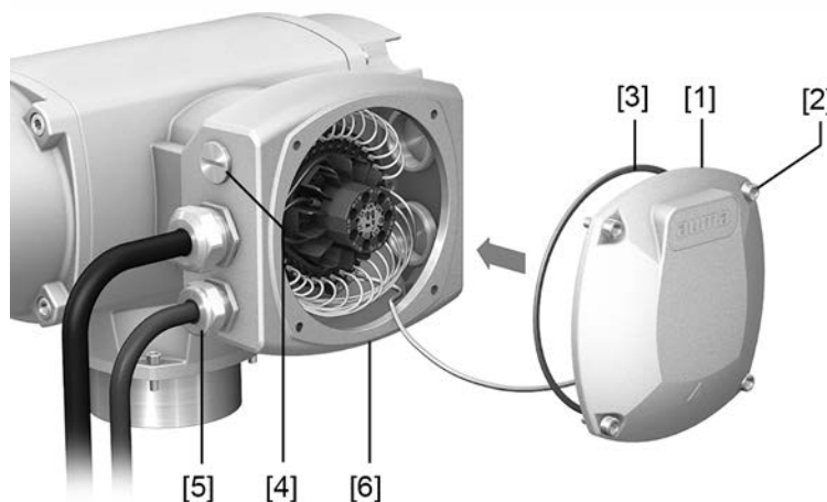
рис. 37: Порядок закрытия отсека контактов
