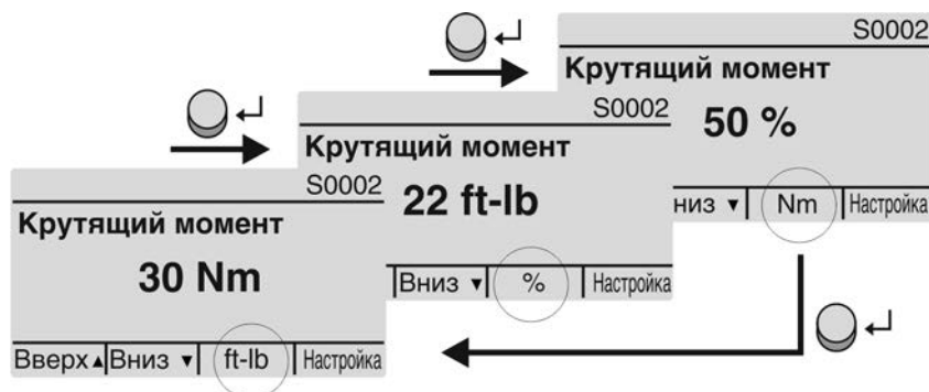
рис. 60: Единицы измерения крутящего момента
