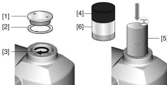
рис. 76: Направление вращения пустотелого вала/штока (в исполнении «с закрытием по часовой стрелке»)
