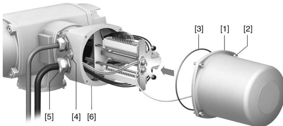
рис. 30: Порядок закрытия отсека контактов
