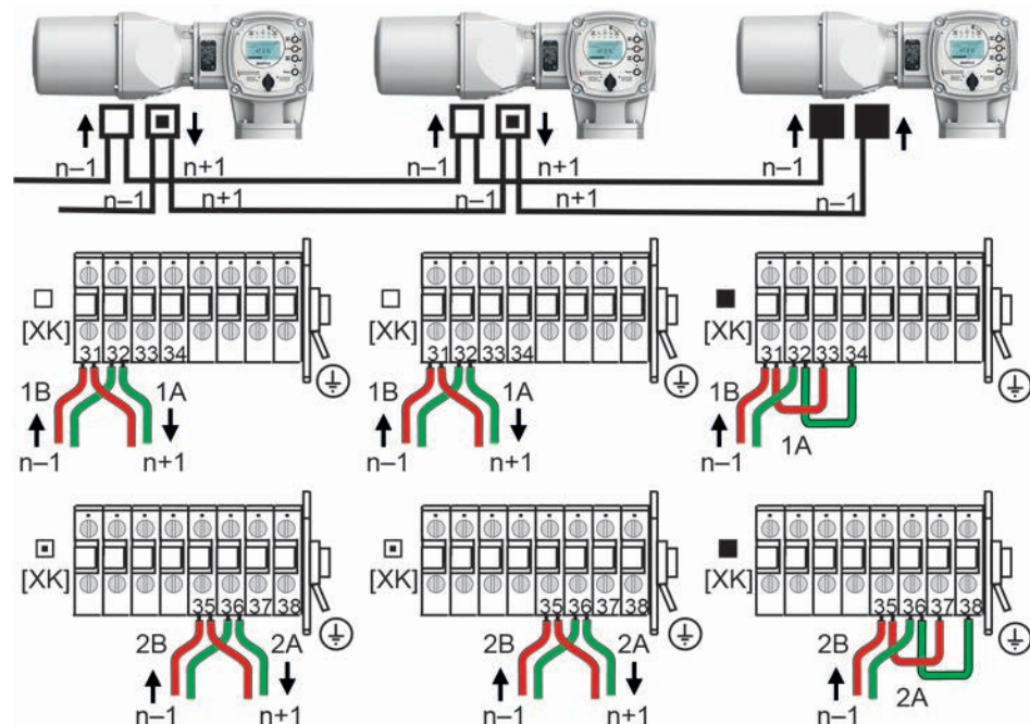
рис. 29: Распределение клемм при линейной топологии (1-канальная или 2-канальная при дублирующей системе I или II)
