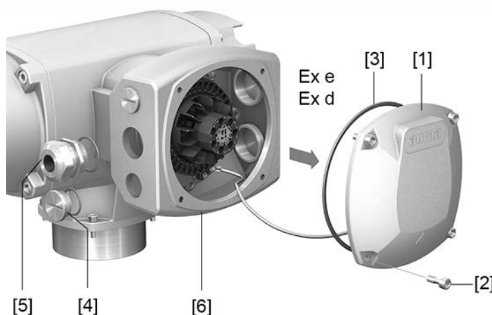
рис. 32: Порядок открытия отсека контактов
