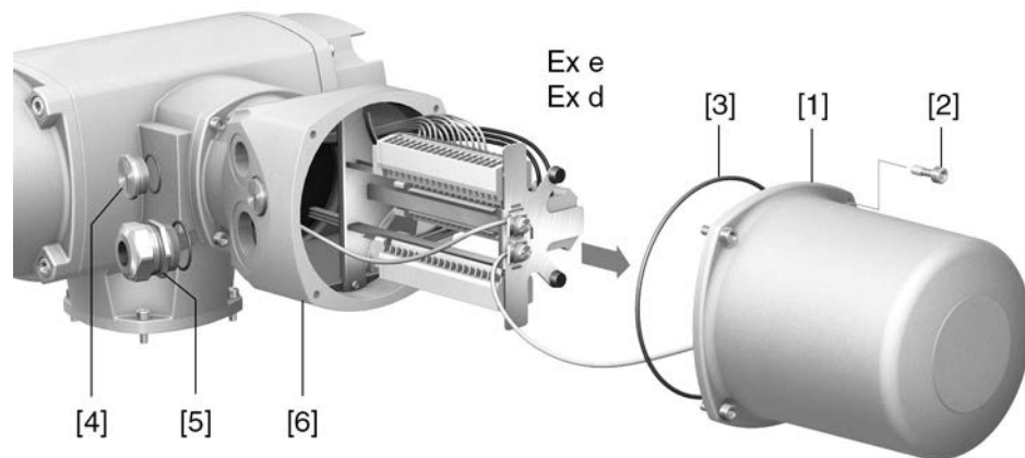
рис. 26: Порядок открытия отсека контактов
