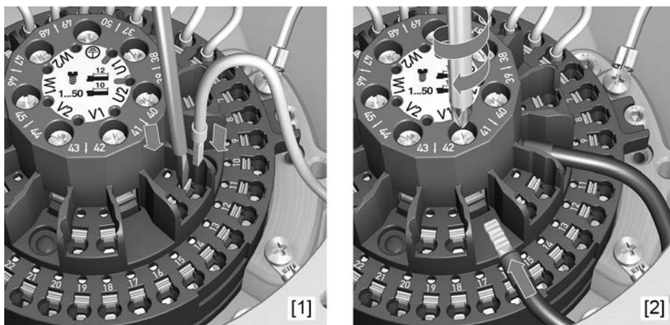
рис. 34: Подключение проводов к блоку зажимов
