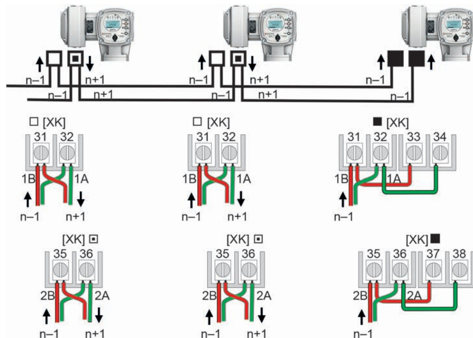
рис. 36: Назначение клемм при линейной топологии (1-канальное или 2-канальное при резервировании AUMA I или II)
