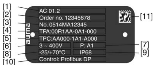
рис. 3: Заводская табличка блока управления электроприводом (пример)
