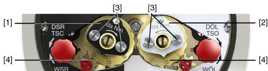
рис. 59: Измерительная головка крутящего момента
