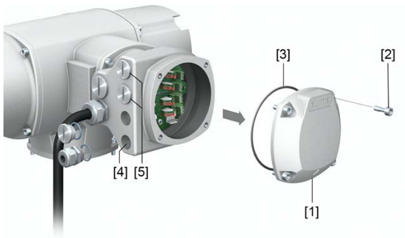
рис. 20: Открытие крышки разъема полевой шины
