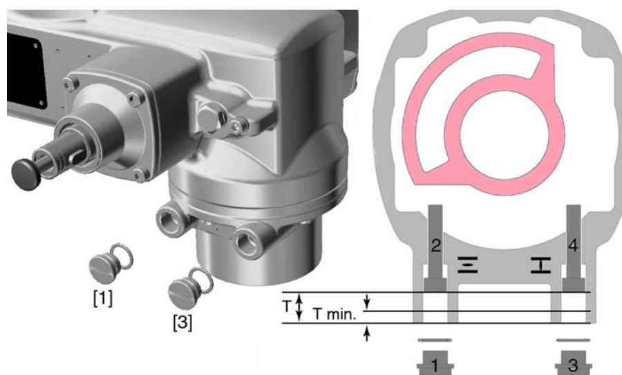
рис. 58: Концевой упор
