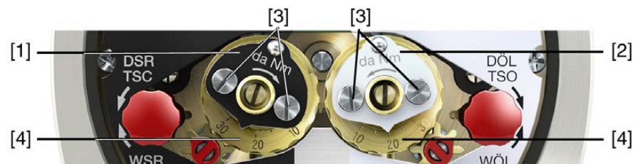
рис. 55: Измерительная головка крутящего момента
