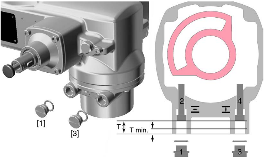
рис. 54: Концевой упор
