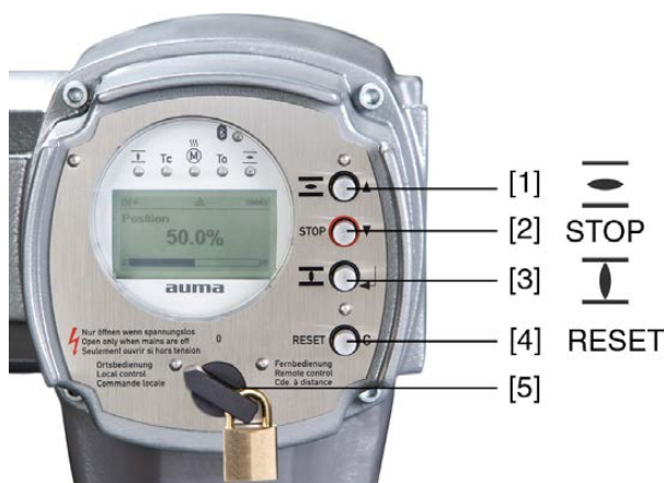
рис. 24: Панель местного управления
