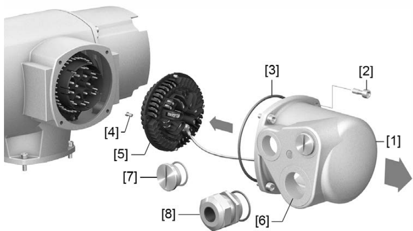
рис. 16: Порядок открытия отсека контактов
