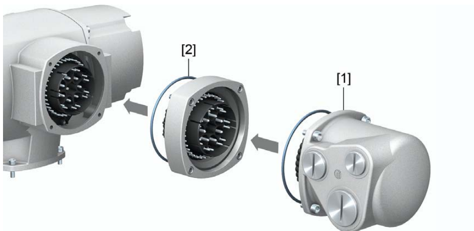
рис. 22: Электрическое подключение с промежуточной рамкой
