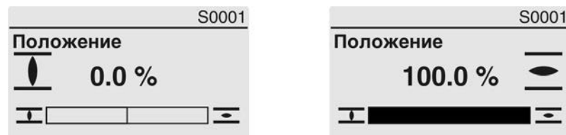
рис. 38: Достигнуто конечное положение ОТКРЫТО/ЗАКРЫТО
