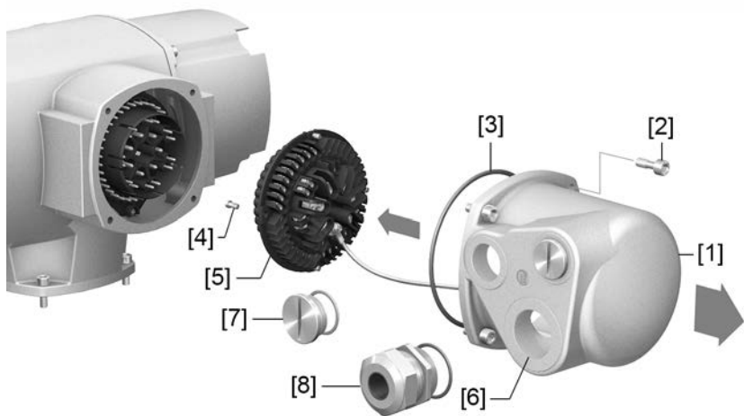
рис. 16: Порядок открытия отсека контактов
