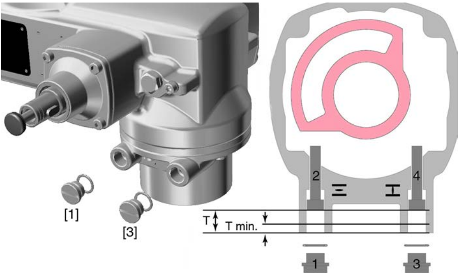
рис. 55: Концевой упор
