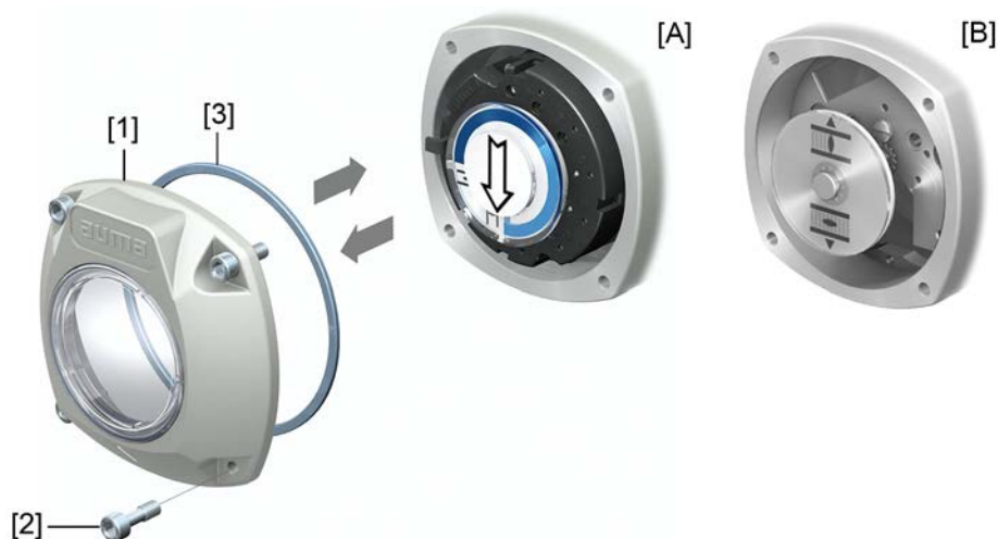
рис. 60: Снятие/установка крышки отсека выключателей
