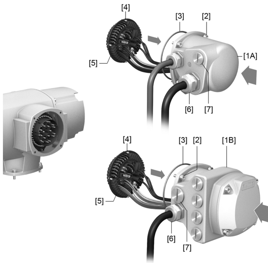
рис. 19: Порядок закрытия отсека контактов
