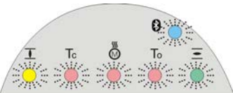
рис. 35: Проверка ламп
