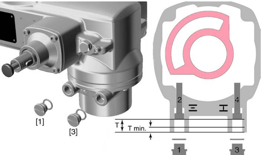
рис. 59: Концевой упор
