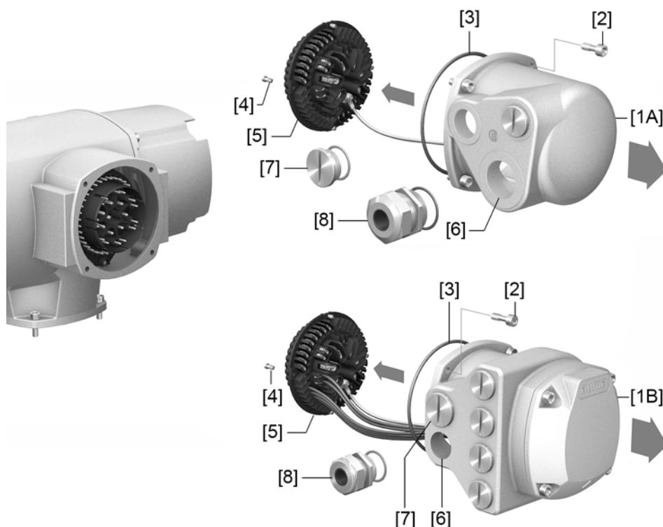
рис. 16: Порядок открытия отсека контактов
