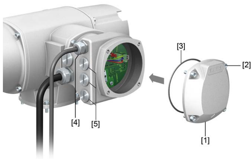
рис. 23: Порядок закрытия отсека контактов HART
