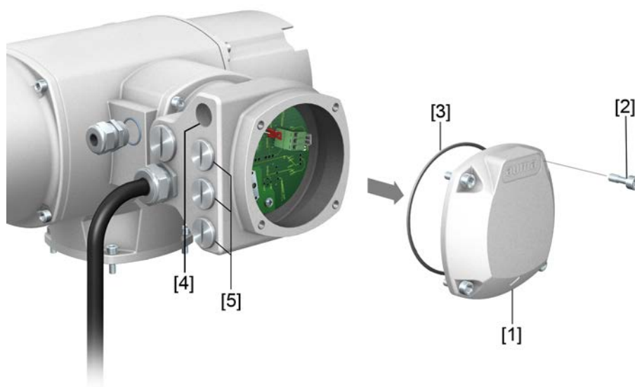
рис. 20: Порядок открытия крышки отсека контактов HART
