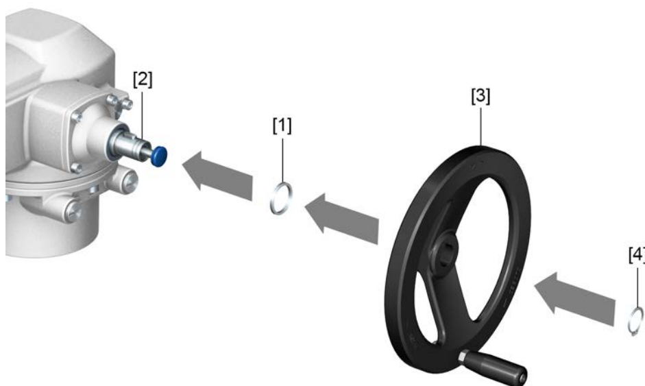
рис. 8: Маховик
