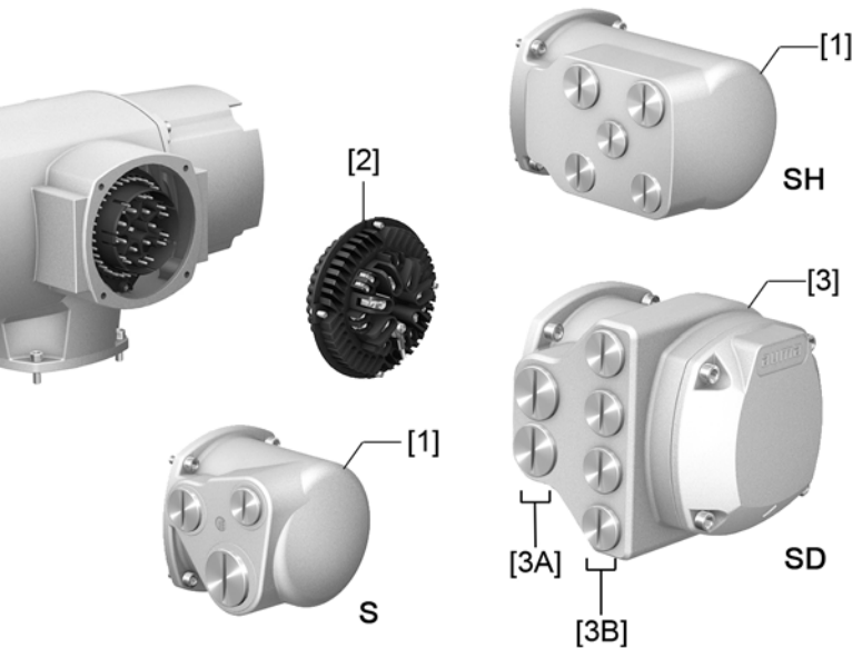
рис. 15: Электрический разъем S, SH и SD
