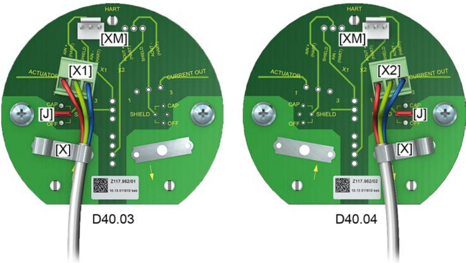
рис. 22: Модификации соединительных плат HART
