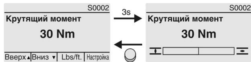
рис. 43: Крутящий момент
