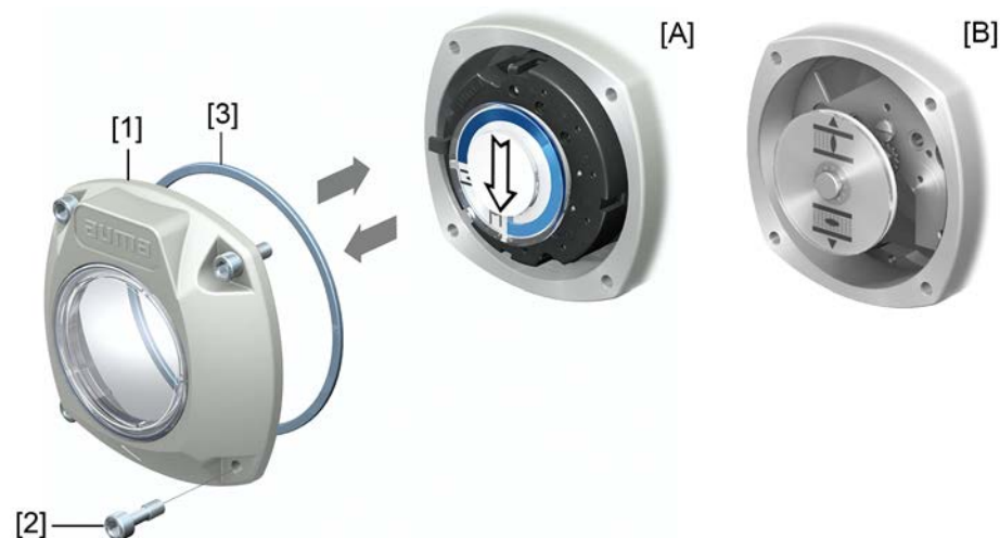
рис. 80: Снятие/установка крышки отсека выключателей
