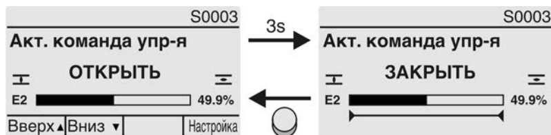
рис. 62: Индикация исполнительных команд ОТКРЫТЬ - ЗАКРЫТЬ
