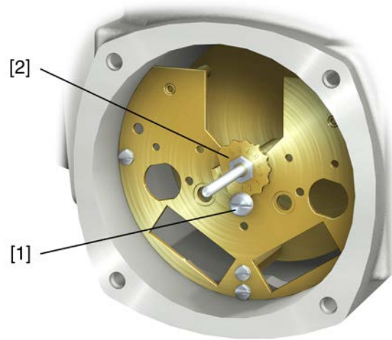
рис. 86: Блок управления с согласующим редуктором
