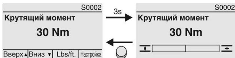
рис. 60: Крутящий момент
