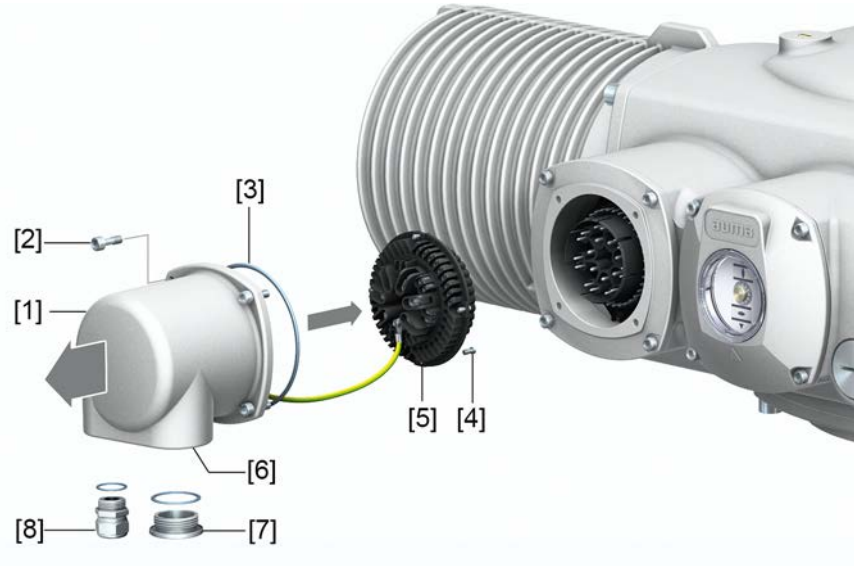
рис. 32: Порядок открытия отсека контактов
